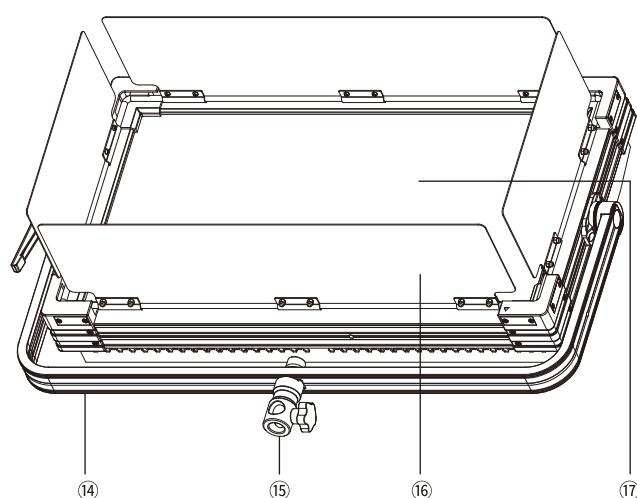
图4 PD-H300B正面视图
