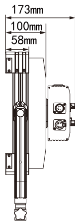
图1 PD-H300B尺寸图(侧面视图)
