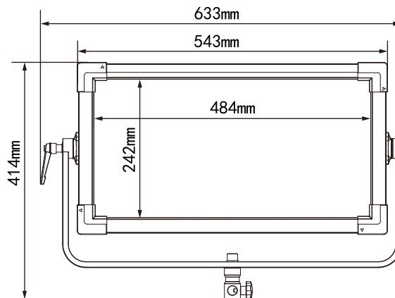
图2 PD-H300B尺寸图(正面视图)
