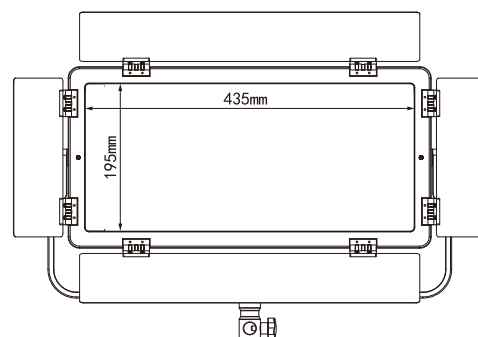
图3 PD-100B正面视图
