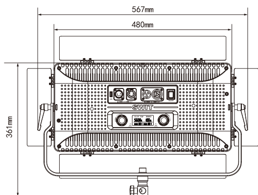
图1 PD-100B背面视图
