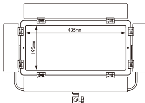
图3 PD-100正面视图
