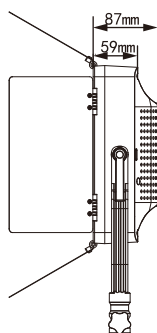
图2 PD-100侧面视图
