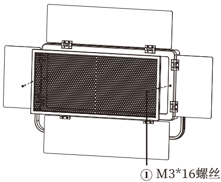
图6 蜂窝安装
