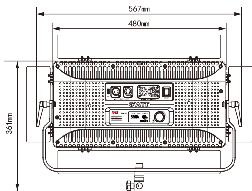
图1 PD-100背面视图
