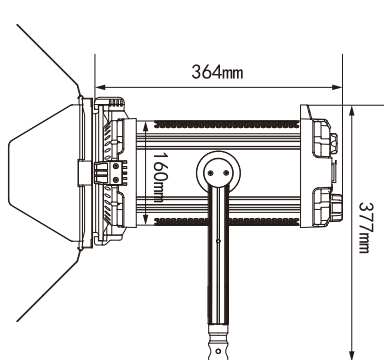
图1 FD-H100侧面视图
