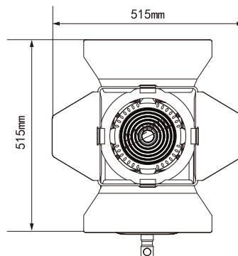
图2 FD-H100正面视图
